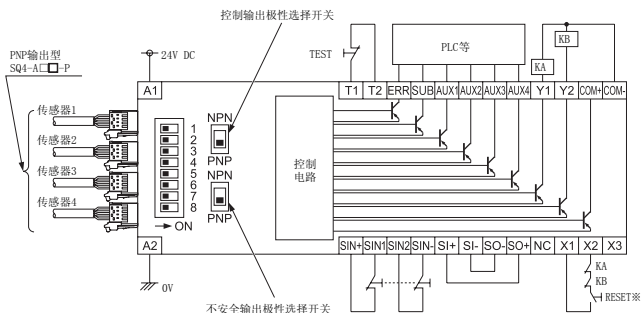
SQ4-C11 控制器
