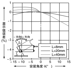
角度特性②
