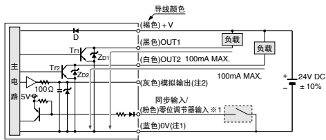
输入、输出电路图
