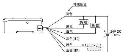
连接图
