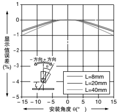
角度特性①
