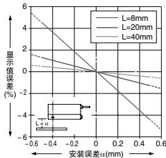
安装误差-显示值误差特性
